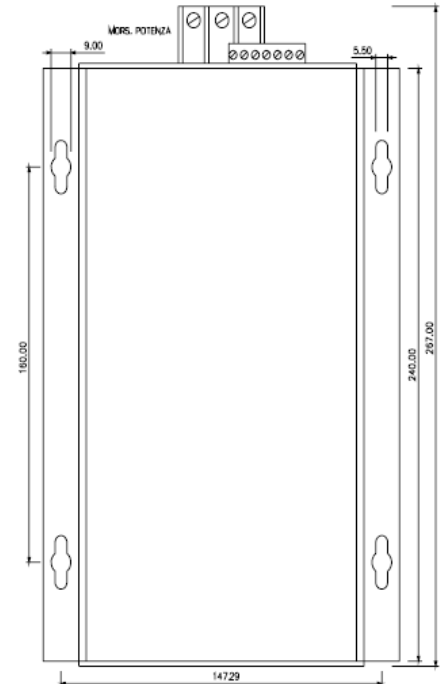
Cod. 100/5 - 100/6 - 100/7 (altezza - Height 165mm)
