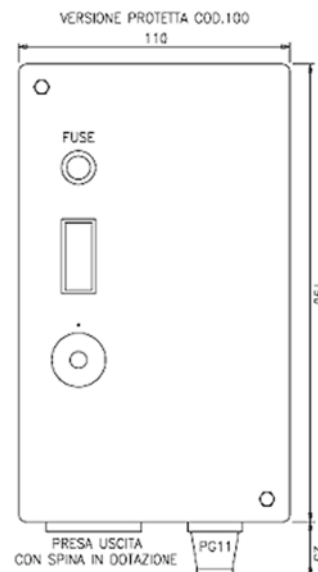
Cod. 100C VERSIONE PROTETTA (altezza - Height 93mm - peso - Weight 660g) 1,2kVA - 220VAC
